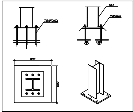
PARTICOLARE ANCORAGGIO TRAVE-PLINTO
